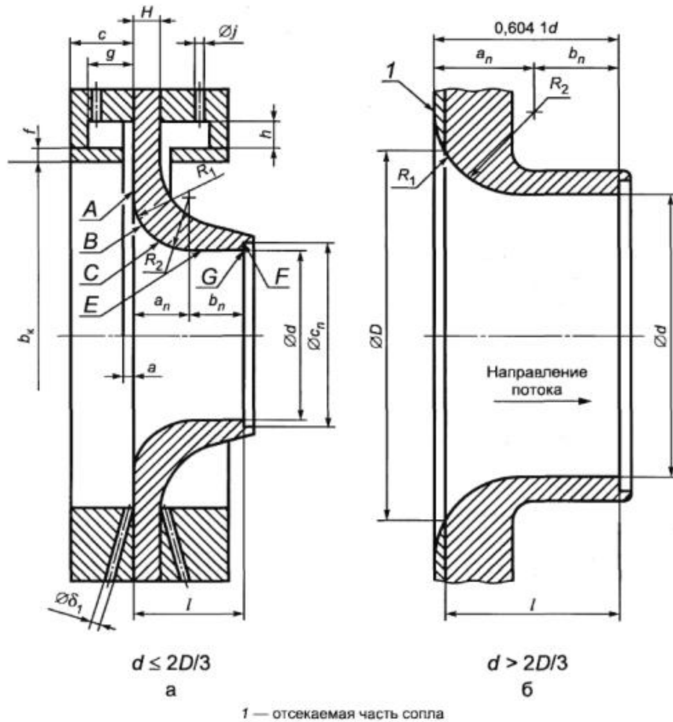
Рисунок 1 - Сопло ИСА 1932
