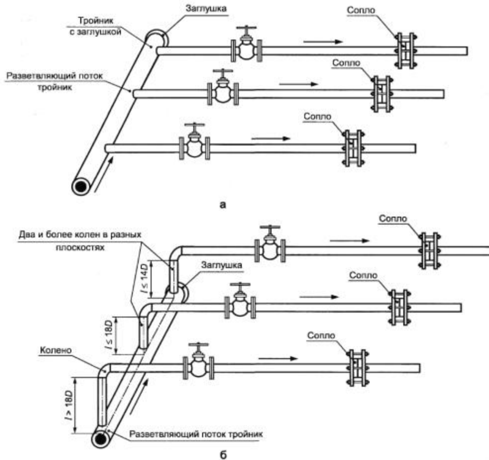
Рисунок 5 - Схемы коллектора
