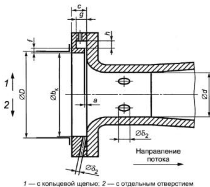
Рисунок 4 - Способы отбора давления, используемые для сопел Вентури
