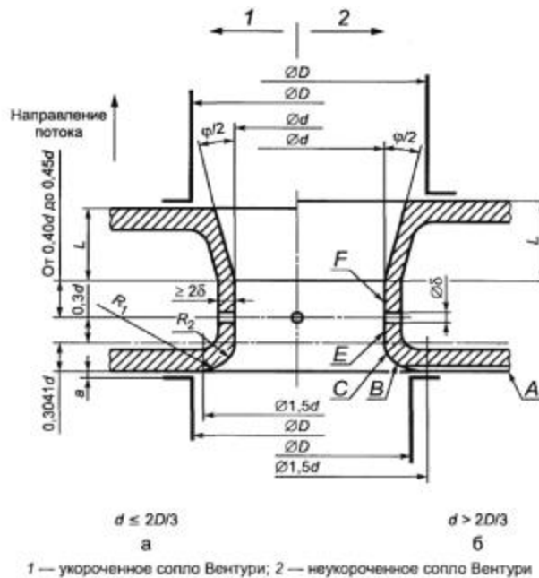
Рисунок 3 - Сопла Вентури
