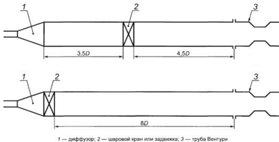
Рисунок 2 - Схема, расположения шарового крана или задвижки при p = 0,6
