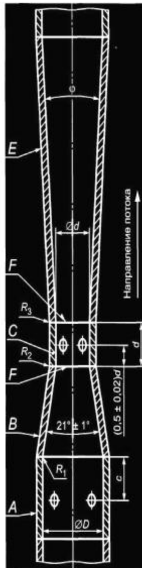
E — диффузор; C — горловина; B — сужающаяся коническая часть; A — входной цилиндрический участок; F — плоскости соединения элементов трубы Вентури; c — см. 5.4.7
